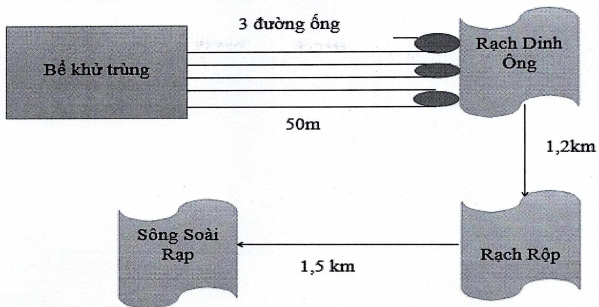
Hình 2. 4 Sơ đồ hệ thống dẫn nước thải sau xử lý ra nguồn tiếp nhận của Nhà máy XLNTTT KCN Hiệp Phước GĐ 1
