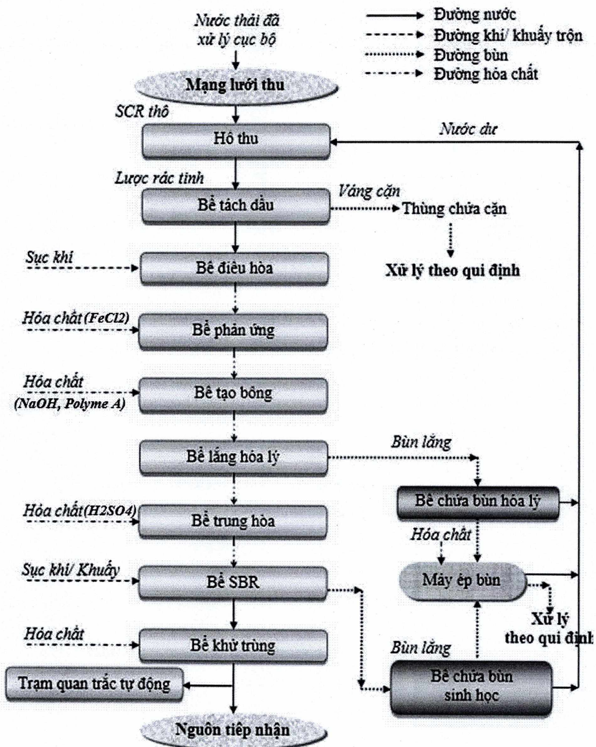
Hình 2. 7 Sơ đồ công nghệ XLNT của Module 2 Nhà máy XLNTTT KCN Hiệp Phước - GD 2
